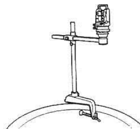
Konzola na šachtu pro teodolit model 3
